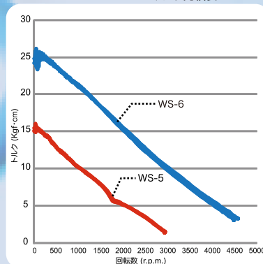
WS-5とWS-6のトルク比較表
