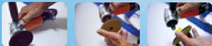
①ロックボタンを押し込み ②パッドを反時計回りに回転 ③スパナを使わず取り外し
