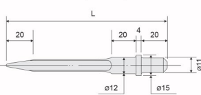
平型 (Flat Chisel) AC No. G-2 シリーズ (Series)
