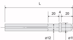
ブランク (Blank Chisel) AC No. G-1 シリーズ (Series)
