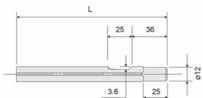
ブランク (Blank Chisel) AC No. F-1 シリーズ (Series)
