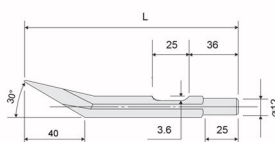
平曲り型 (Flux Chisel) AC No. F-3 シリーズ (Series)
